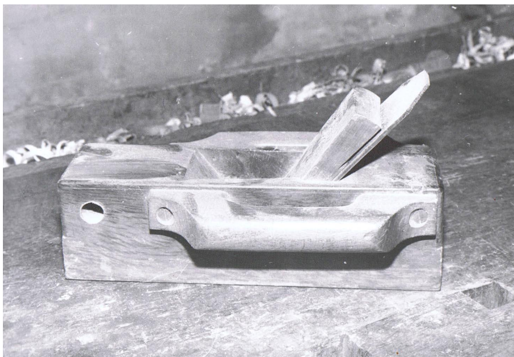
Rabot à deux mains soit galère selon JFR.
