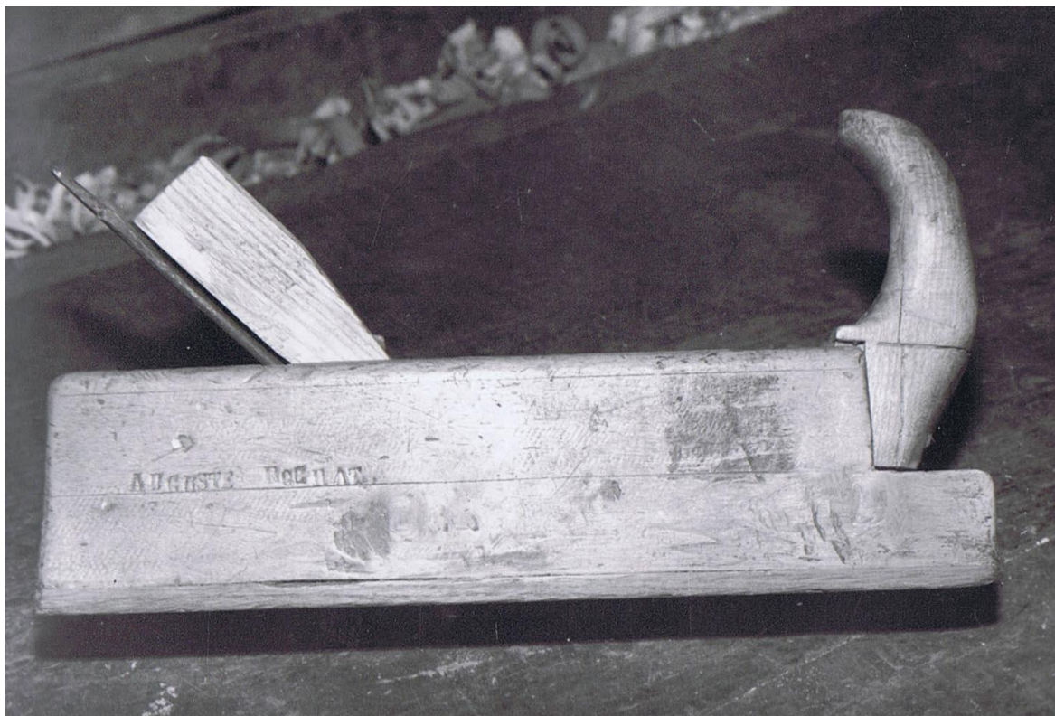
Rabot à raplanir.
