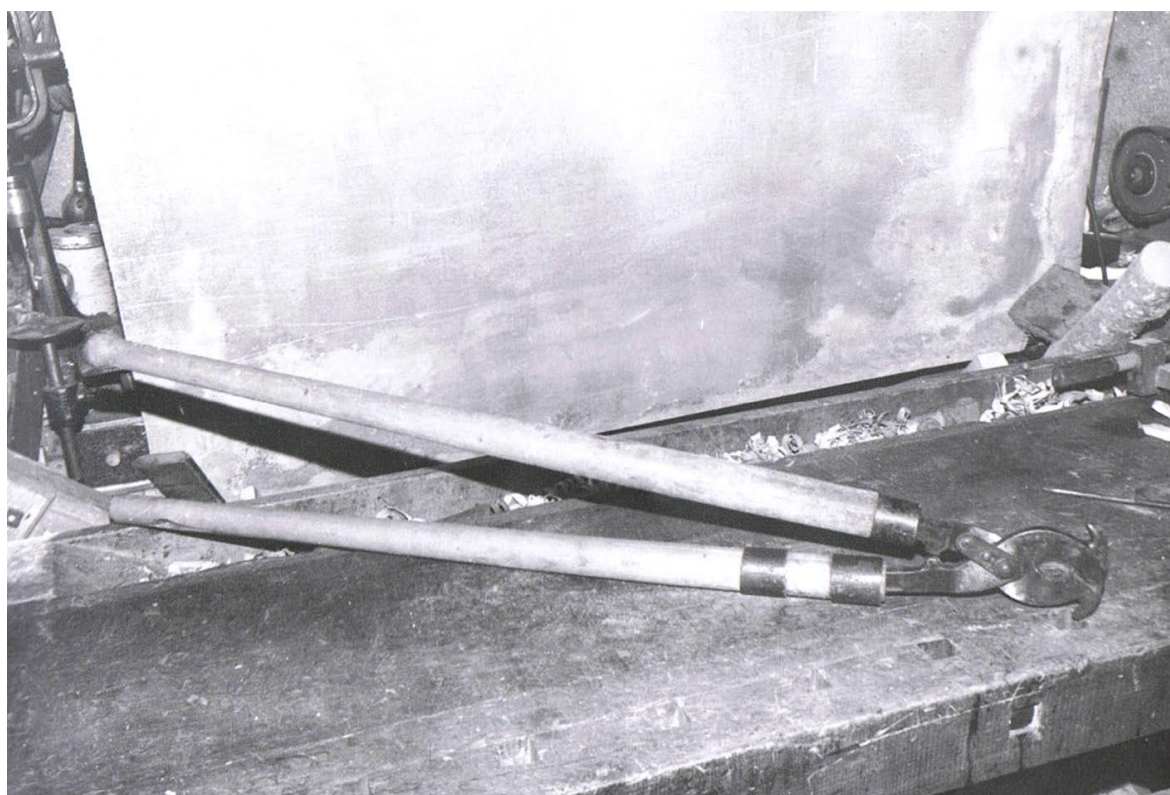
La cisaille à couper les noisetiers.
