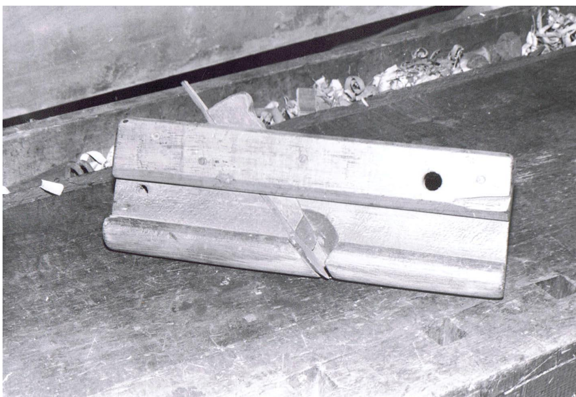
Rabots à chanfrein.
