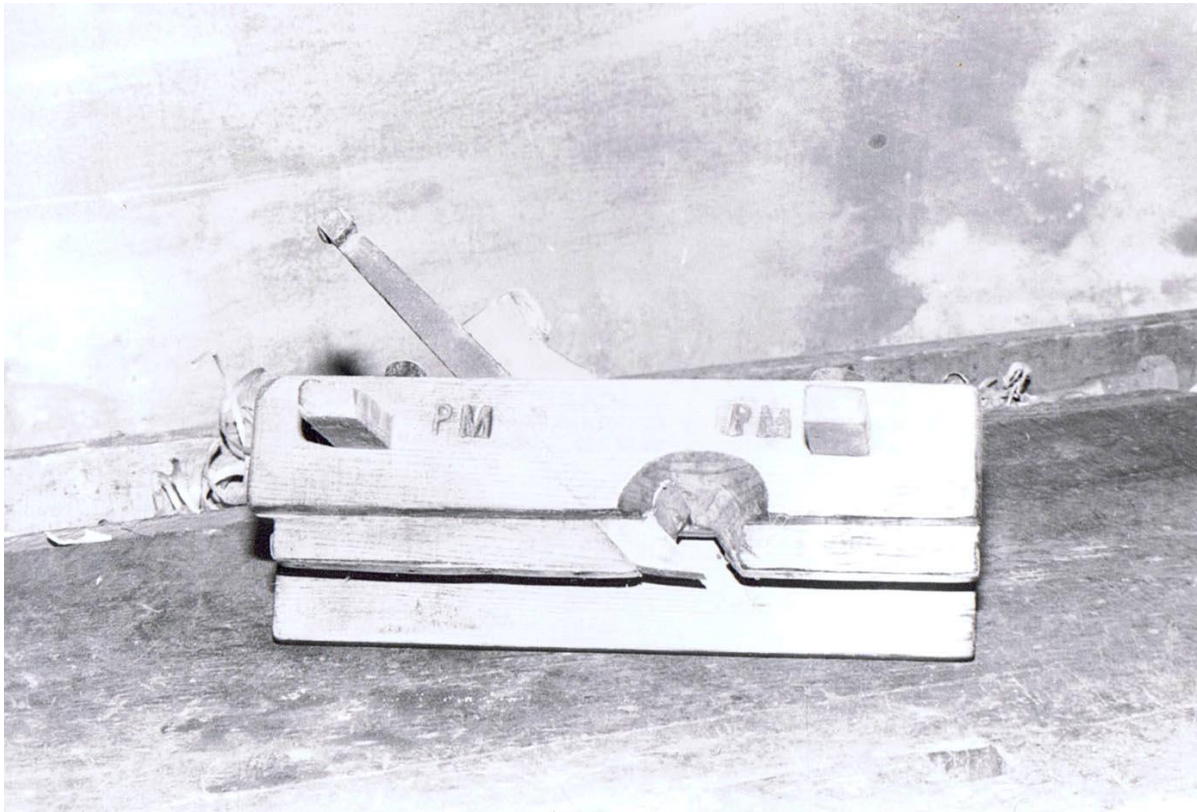
Rabot à chanfrein.
