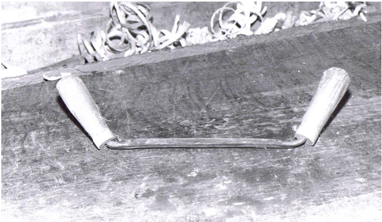
Le couteau à deux mains pour éparer.
