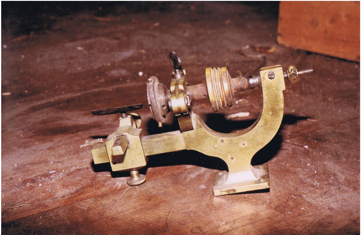
Un petit tour d'horloger, qui prouve que là aussi, malgré que l'on fut essentiellement agricole, l'on pratiqua la petite industrie.
